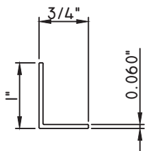
3/4\"X1\" ANGLE MW13177
