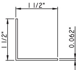
1 1/2\"X1 1/2\" ANGLE M13416
