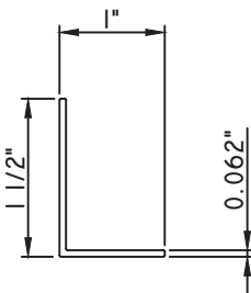
1\"X1 1/2\" ANGLE MAX4050
