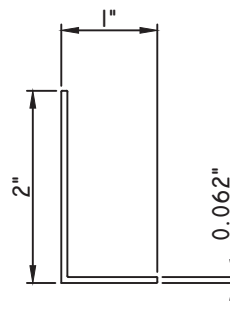
1\"X2\" ANGLE MW10726
