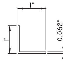
1\"X1\" ANGLE MW1667
