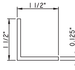
1 1/2\"X1 1/2\" ANGLE MW4220
