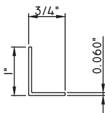
3/4"X1" ANGLE MW13177
