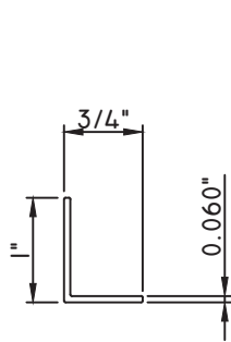
3/4"X1" ANGLE MW13177
