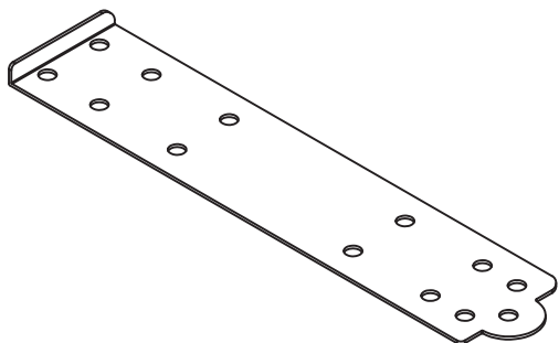
7" MASONRY CLIP LW7007 BENT 9" MASONRY CLIP LW7009 BENT
