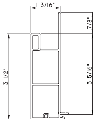
BRICKMOLD W/FIN WN2376
