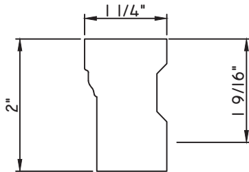
COMPOSITE BRICKMOLD GOSSEN_635 COMP-BM
